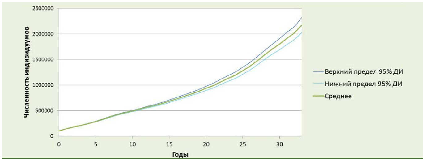
Рисунок 3. Динамика численности популяции сайгака при добавлении в модель ежегодного осеннего промысла (среднее за 100 прогонов).
